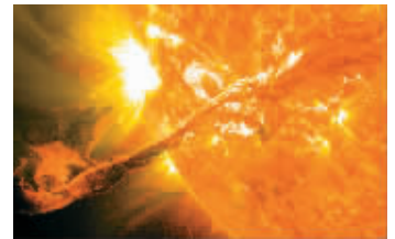
2012年8月31日,SDO拍摄下的太阳爆发日珥照片。
